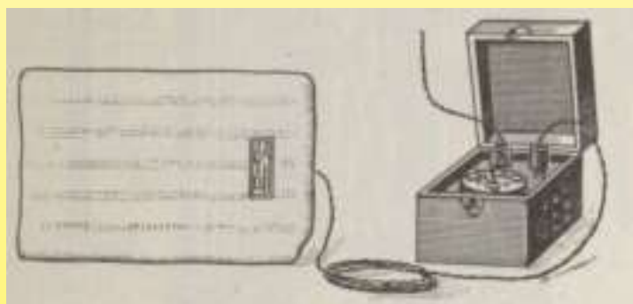
‘Thermoplasme Parvillée’ 1903. Размеры 25 см x 35 см Мощность: “Меньше, чем у 5 ламп-свечей” или около 50 ватт (на данный момент). Поверхностный заряд составлял около 0,06 Вт/см 2 .
