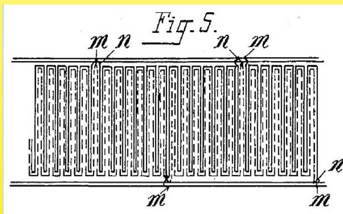
m, n: Детали соединений питающих проводов в отбортовках. Эта техника до сих пор используется в электрической трассировке (запатентована Камилем Эрроттом в 1901 году).
