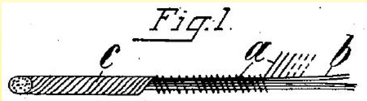
Нагревательный шнур (запатентован Камилем Эрроттом, 1901 г.). А = нагревательный провод; В = текстильный сердечник; С = внешняя обмотка, намотанная в противоположном направлении от нагревательного провода
